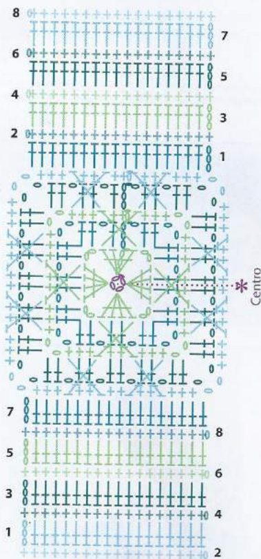
Lateral y base de la capellada
